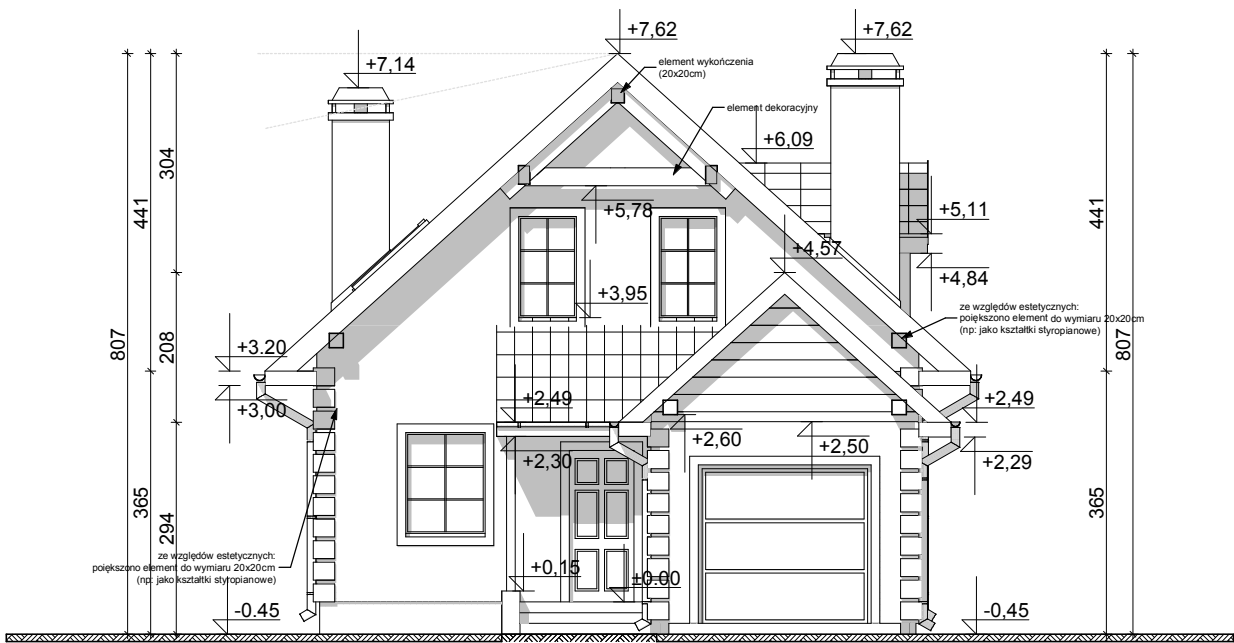
ELEWACJA FRONTOWA
