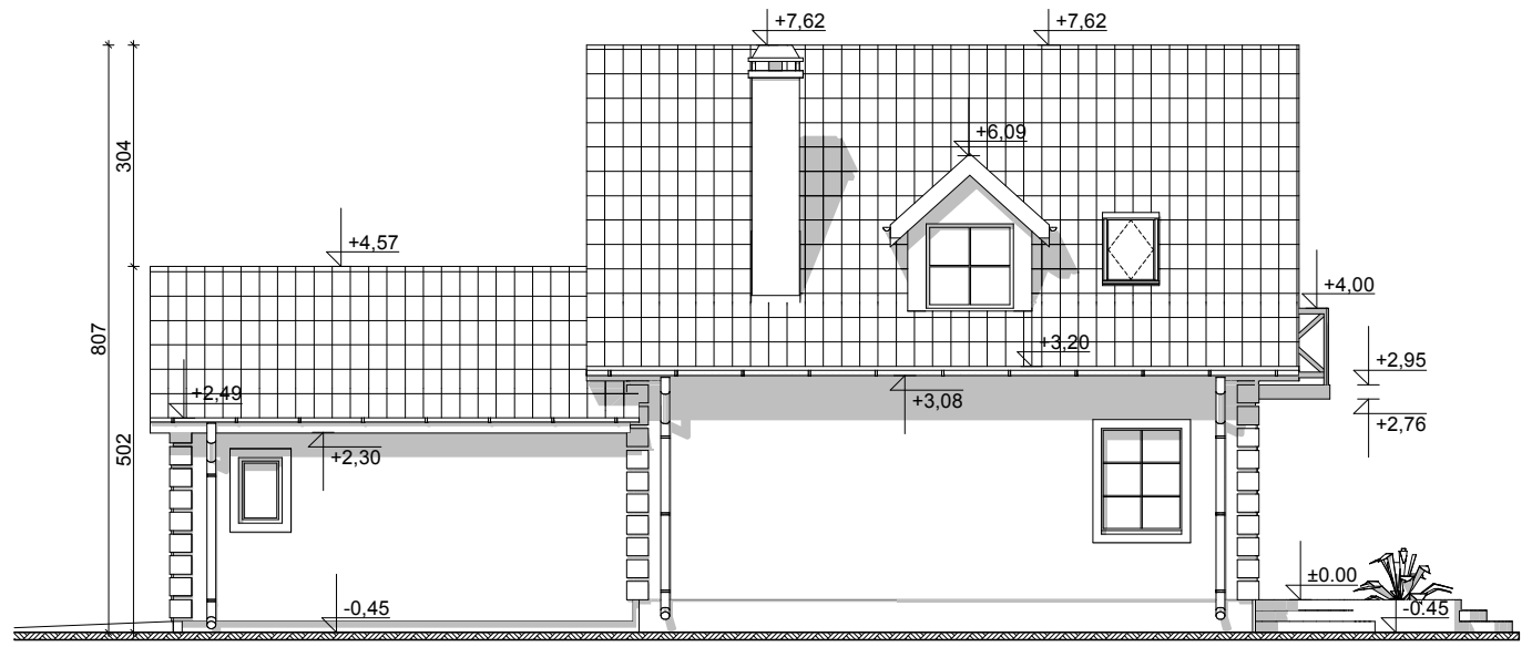
ELEWACJA BOCZNA
