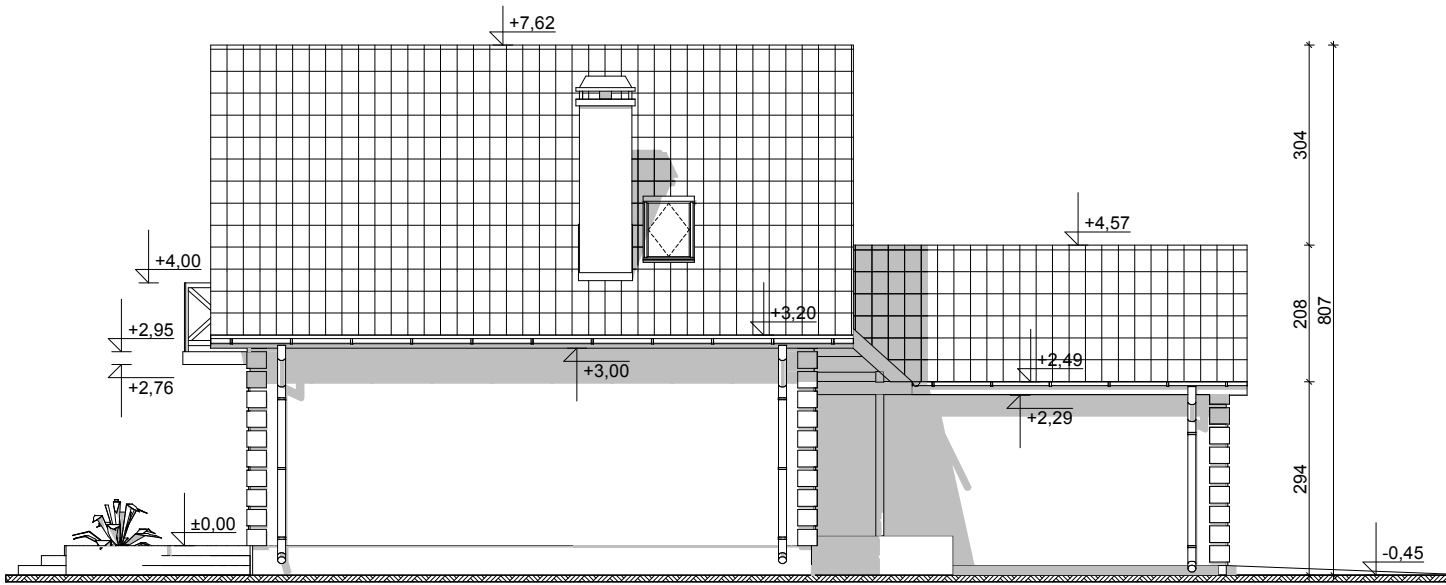
ELEWACJA BOCZNA
