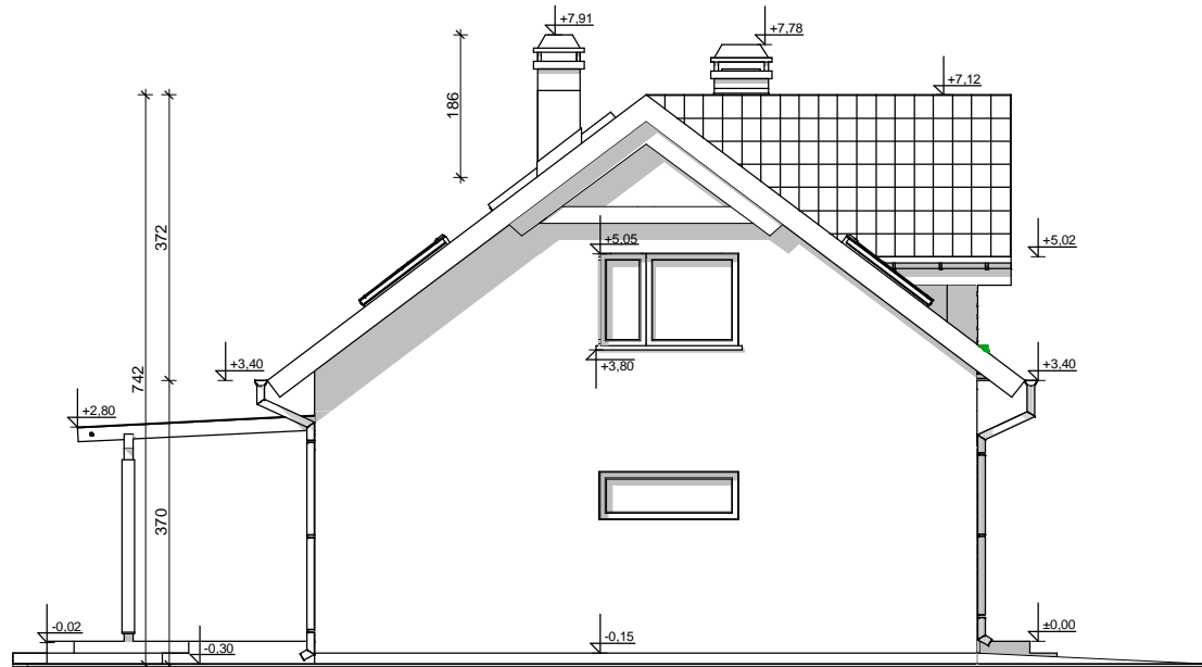
ELEWACJA BOCZNA
