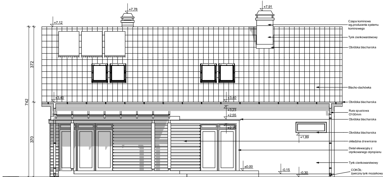
ELEWACJA OGRODOWA
