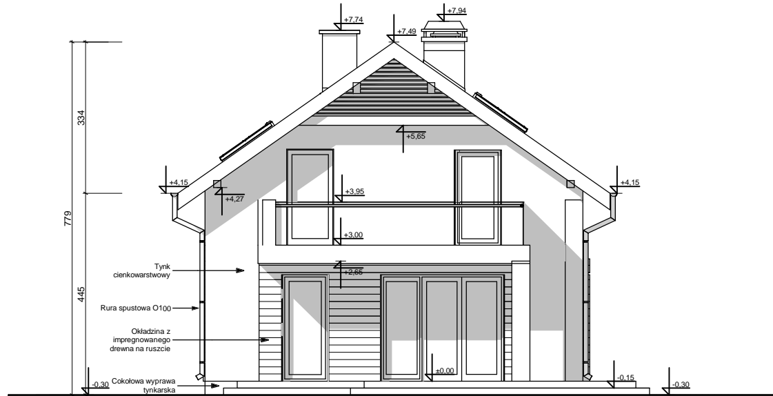
ELEWACJA BOCZNA
