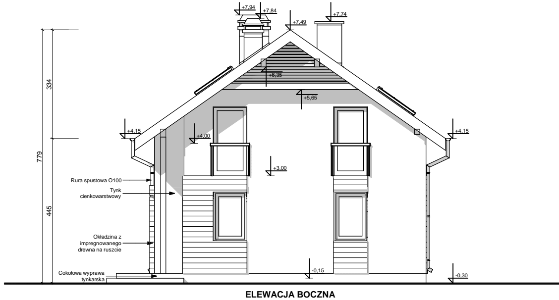
ELEWACJA BOCZNA
