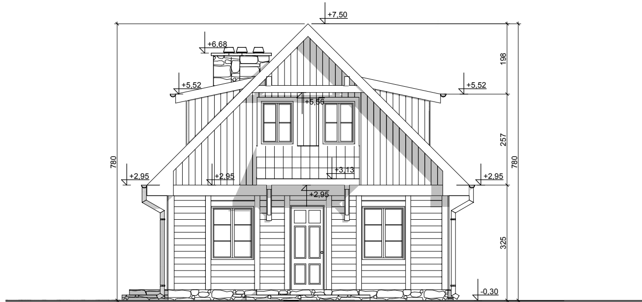
ELEWACJA FRONTOWA
