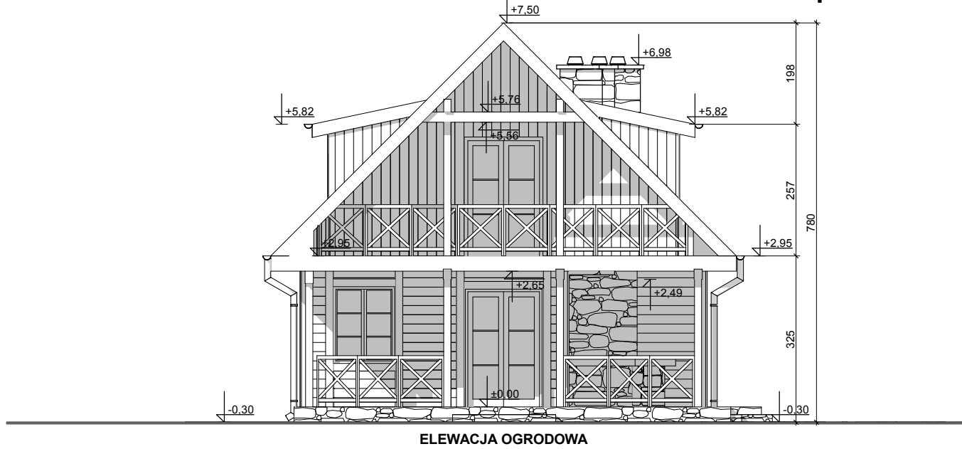
ELEWACJA OGRODOWA
