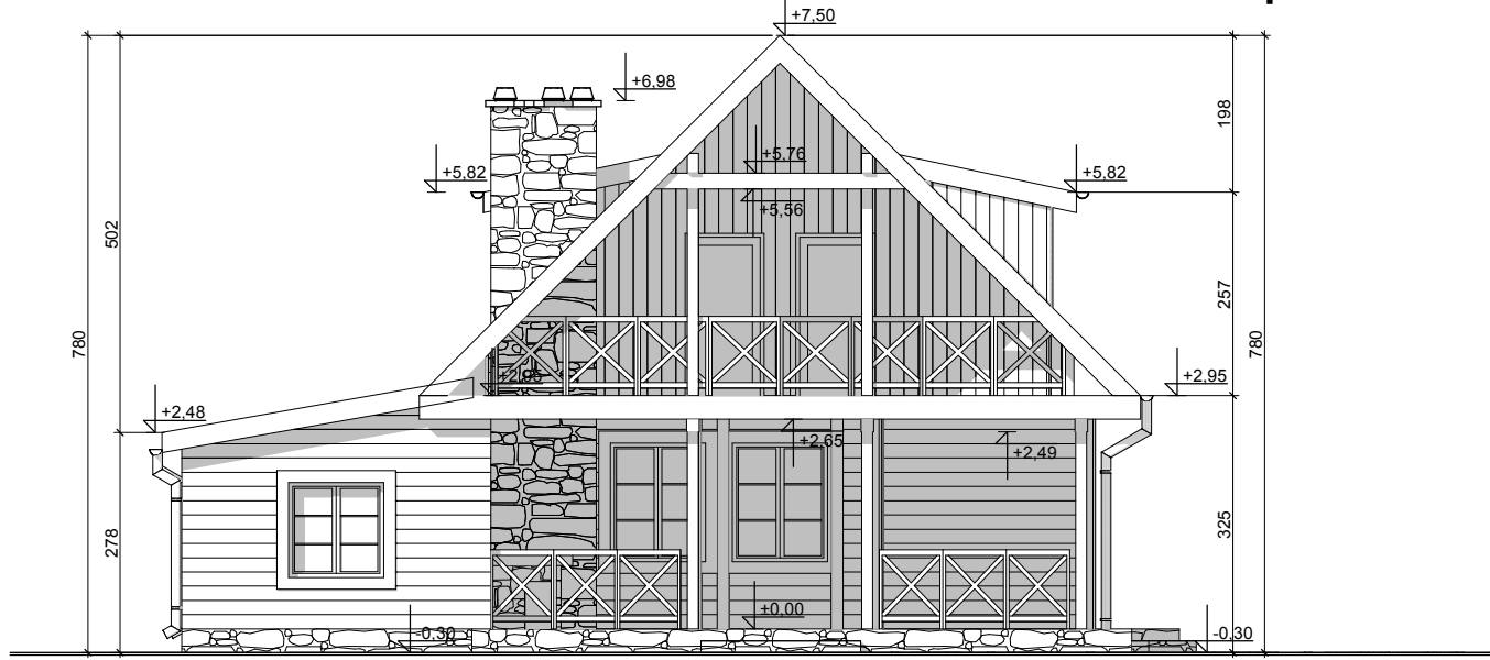
ELEWACJA OGRODOWA
