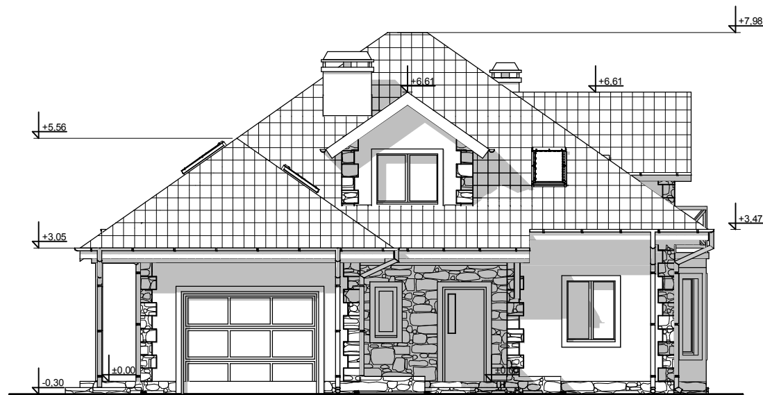
ELEWACJA PÓLNOĆNA
