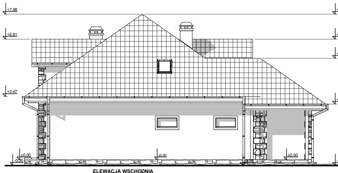
ELEWACJA WSCHODNIA
