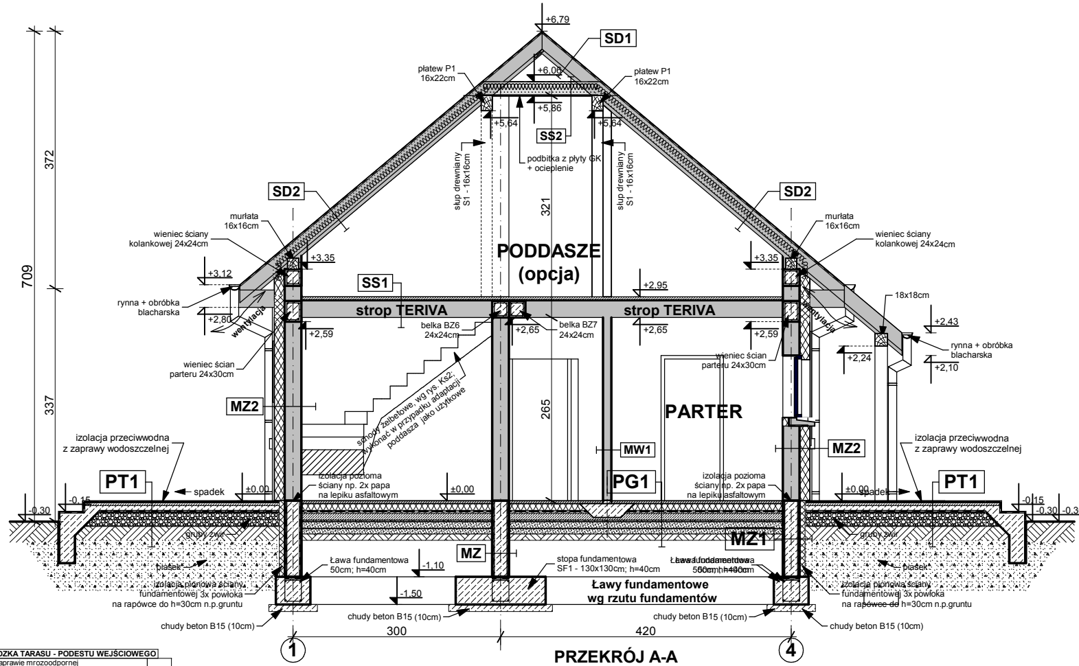
PRZEKRÓJ A-A
