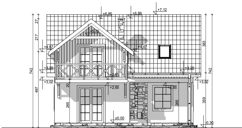
ELEWACJA TYLNA
