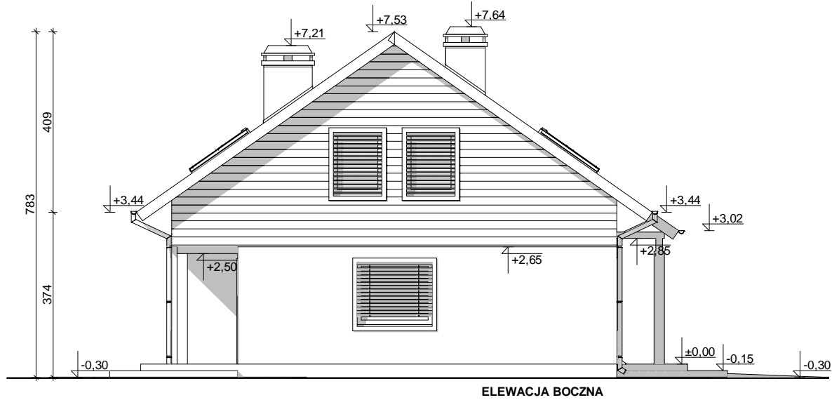
ELEWACJA BOCZNA
