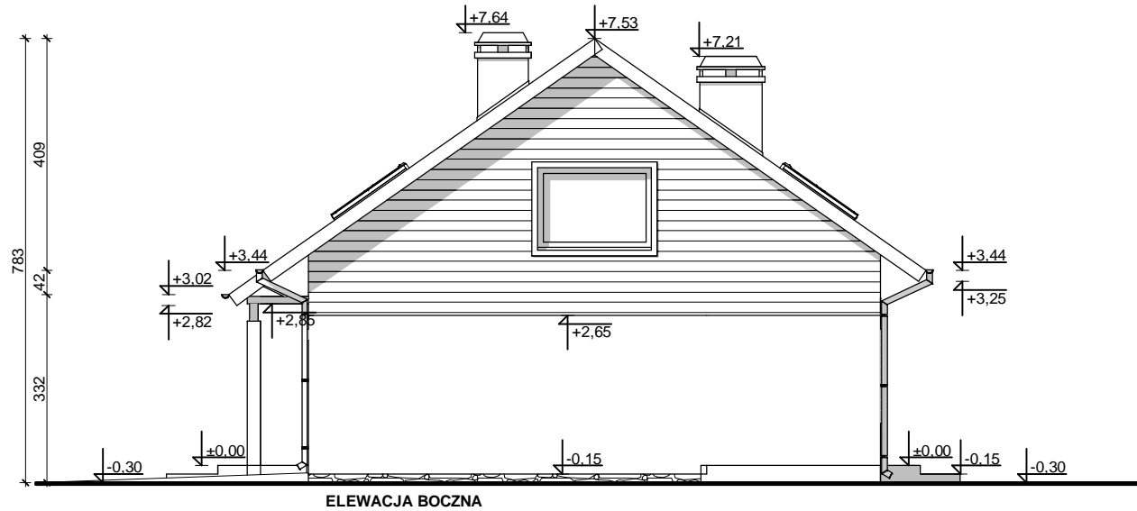
ELEWACJA BOCZNA
